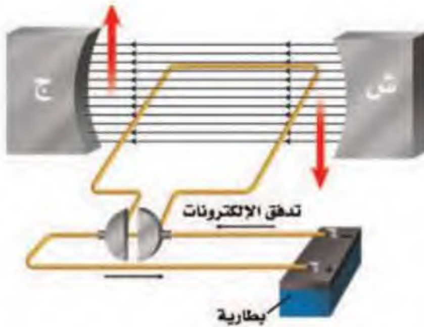
ب. يؤثر المجال المغناطيسي الدائم في الملف بقوة تجعلها تدور حول نفسها، ما دام التيار ماراً فيها.
